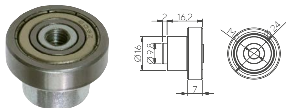
50.18 Cuscinetti Foro M6
