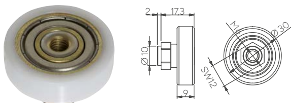
50.18 Cuscinetti Foro M6
