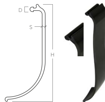
art. 50186516 50186517
