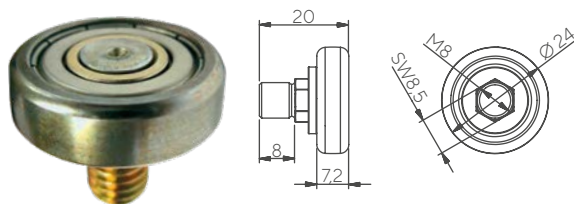
50.18 Cuscinetti Foro M8
