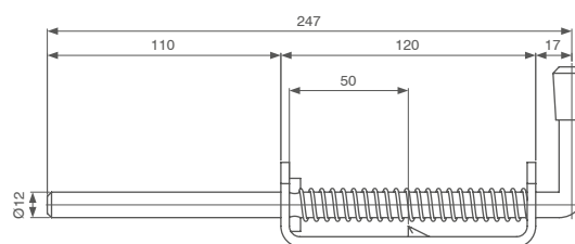
Perno lungo
