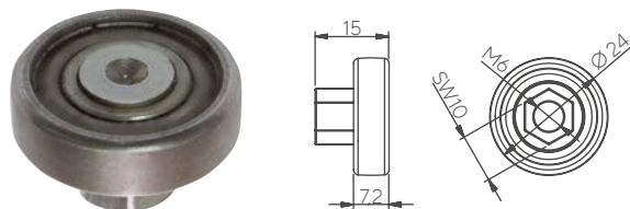
50.18 Cuscinetti Foro M6
