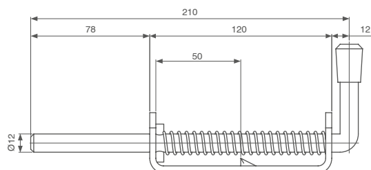
Perno corto
