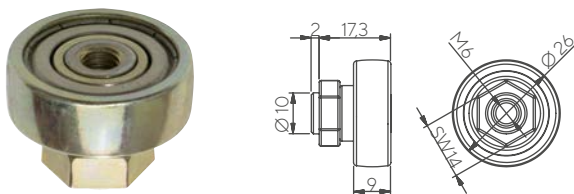
50.18 Cuscinetti Foro M6
